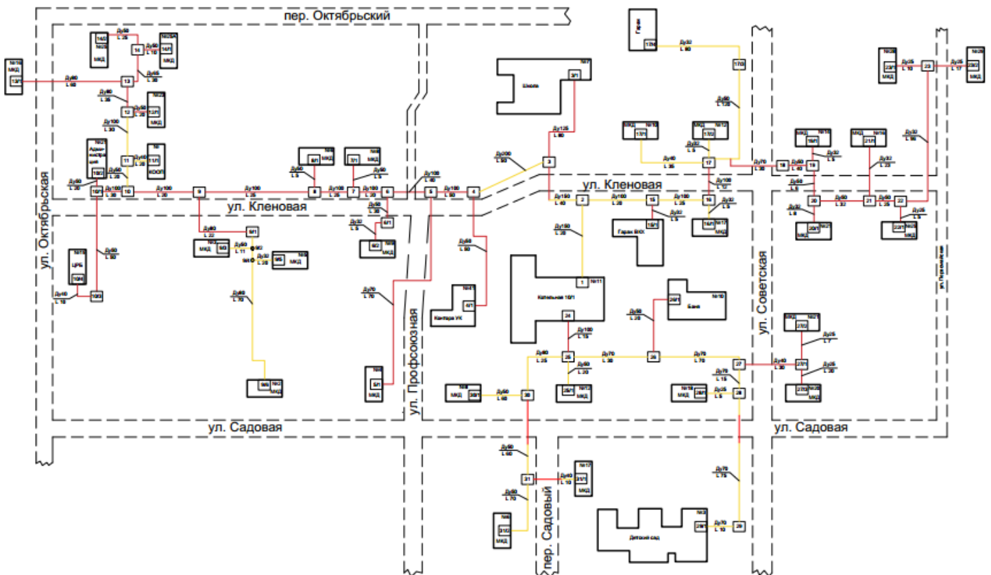
Рисунок 2. Схема теплоснабжения от муниципальной котельной №10/1
